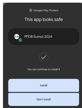
Gambar 9. Install aplikasi
